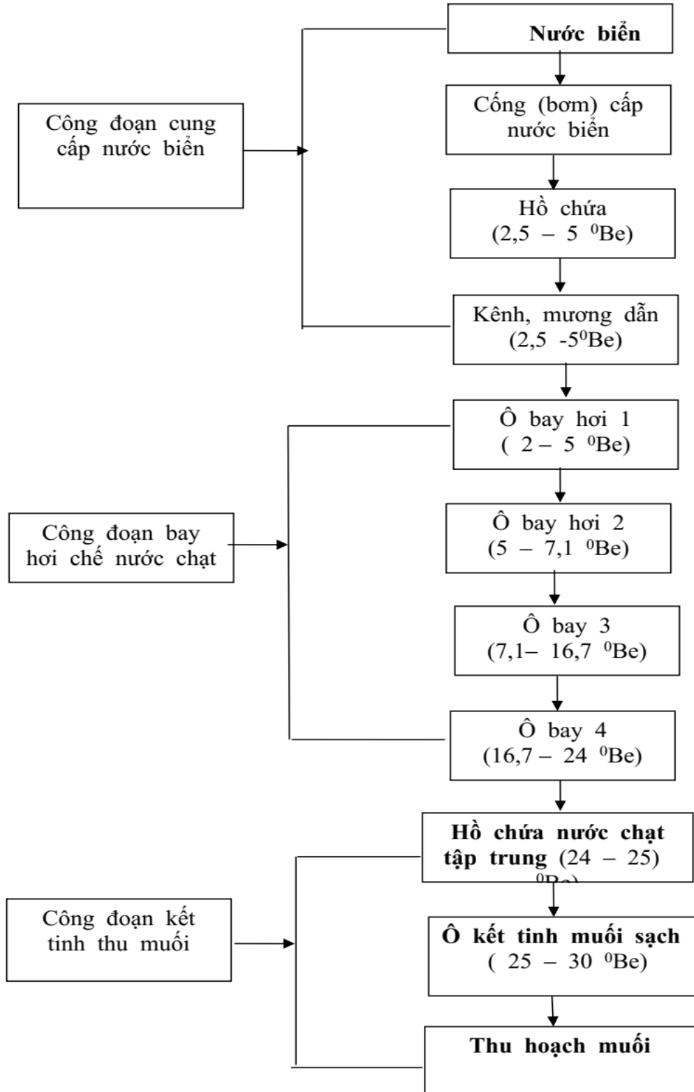
Hình 4. Sơ đồ quy trình công nghệ sản xuất muối sạch phơi nước phân tán
